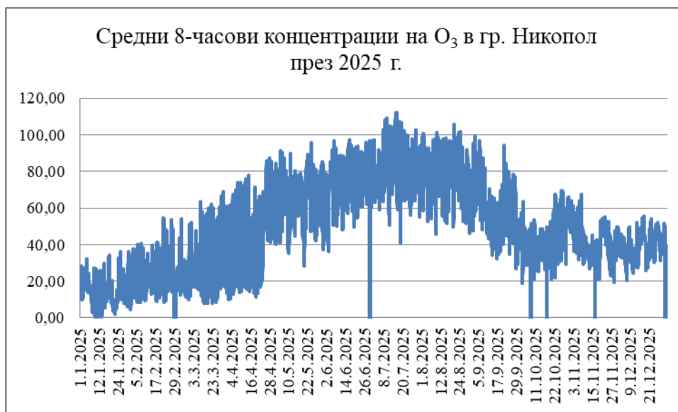
Фиг. 13. Средни 8-часови концентрации на O 3 в гр. Никопол през 2025 г.
